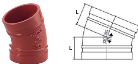
22.5D 엘보
