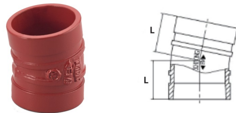
11.25D 엘보
